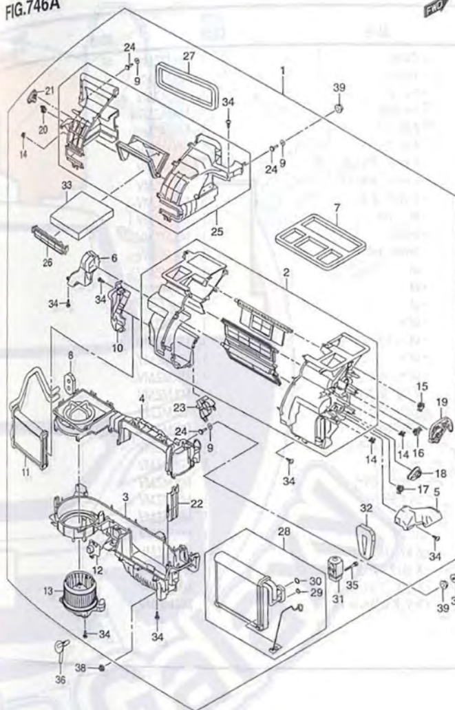
FIG.746A ヒータユニット (G)
